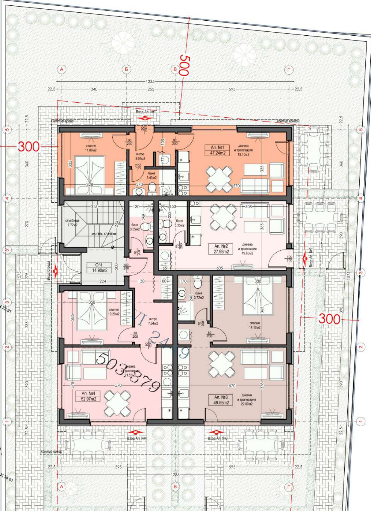
РАЗПРЕДЕЛЕНИЕ 1-ви этаж кота +0.00 М1:100 ЗП 192.65кв.м.
