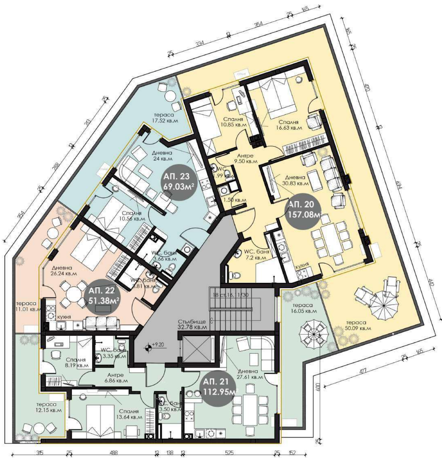
Разпределение на пети етаж
