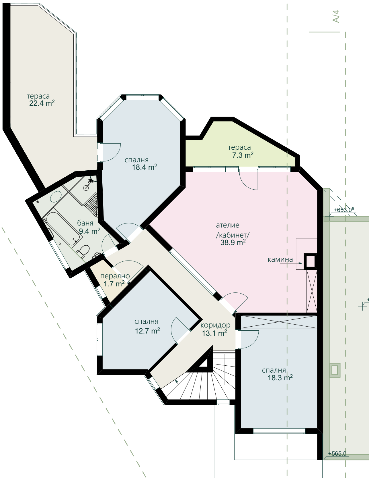
РАЗПРЕДЕЛЕНИЕ ВТОРИ ЕТАЖ М 1:100
