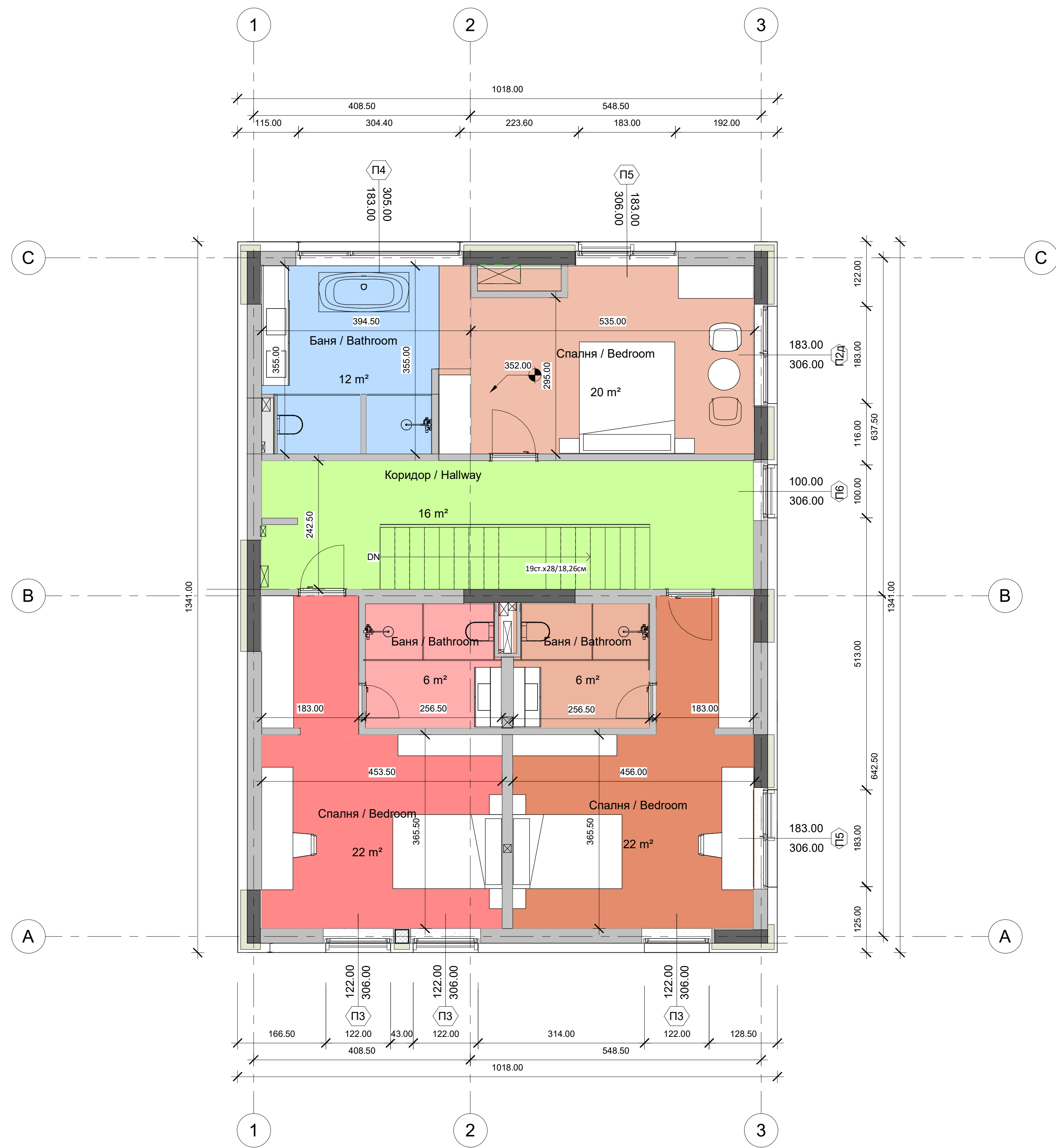
СГРАДА М3 Тип 5/ HOUSE M3 Type 5 НИВО +3.52m / LEVEL +3.52m ЕТАЖ 2 / LEVEL 2
