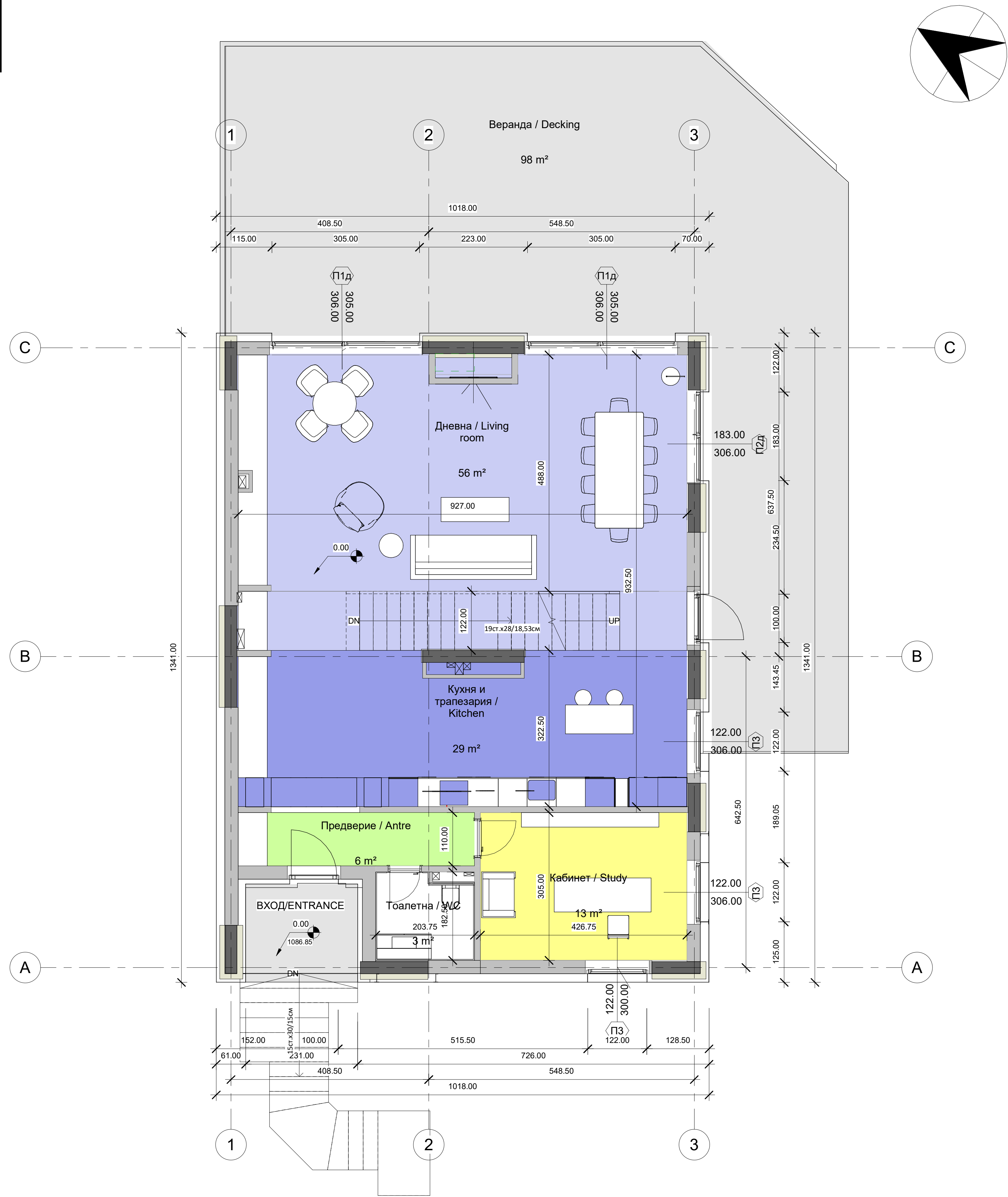
СГРАДА М3 Тип 5 / HOUSE M3 Type 5 НИВО ±0.00m / LEVEL ±0.00m ЕТАЖ 1 / LEVEL 1
