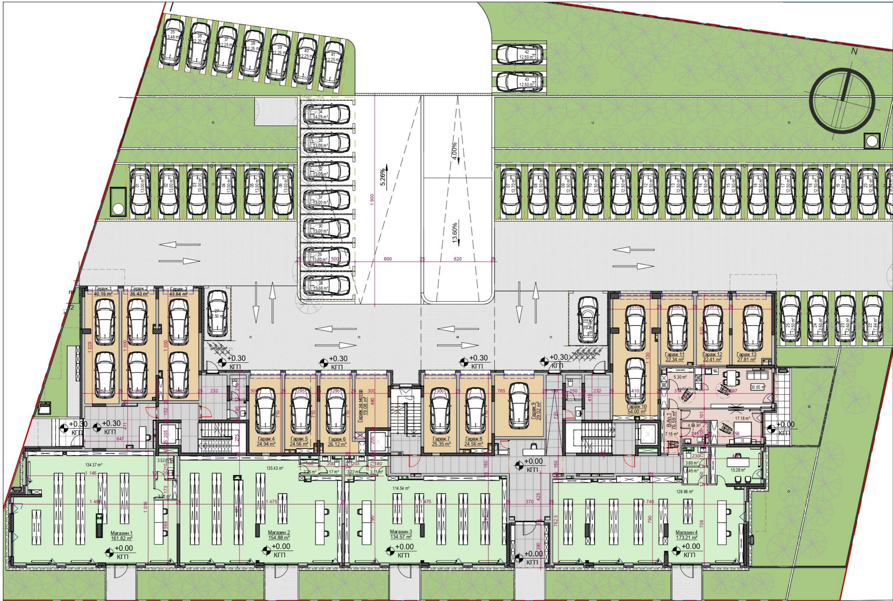
Разпределение партерен етаж кота +0,00
