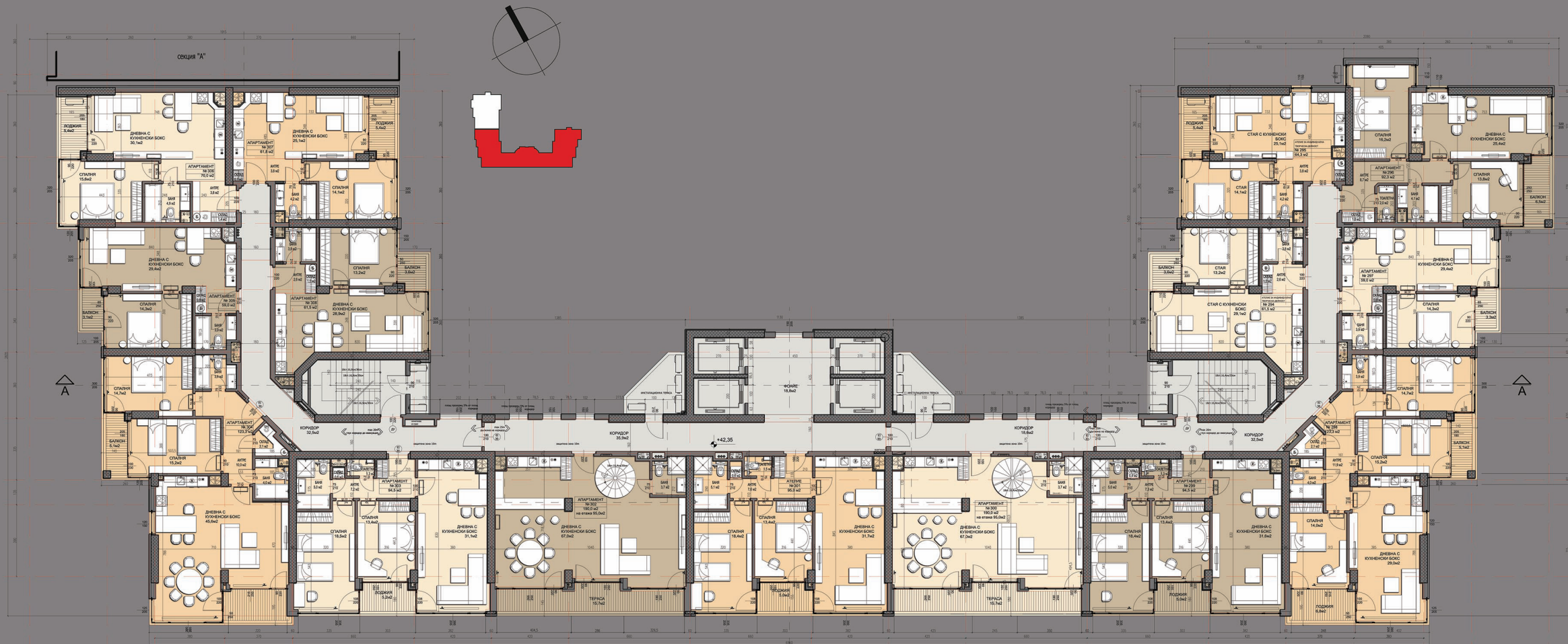
РАЗПРЕДЕЛЕНИЕ 15 ЕТАЖ СЕКЦИЯ Б
