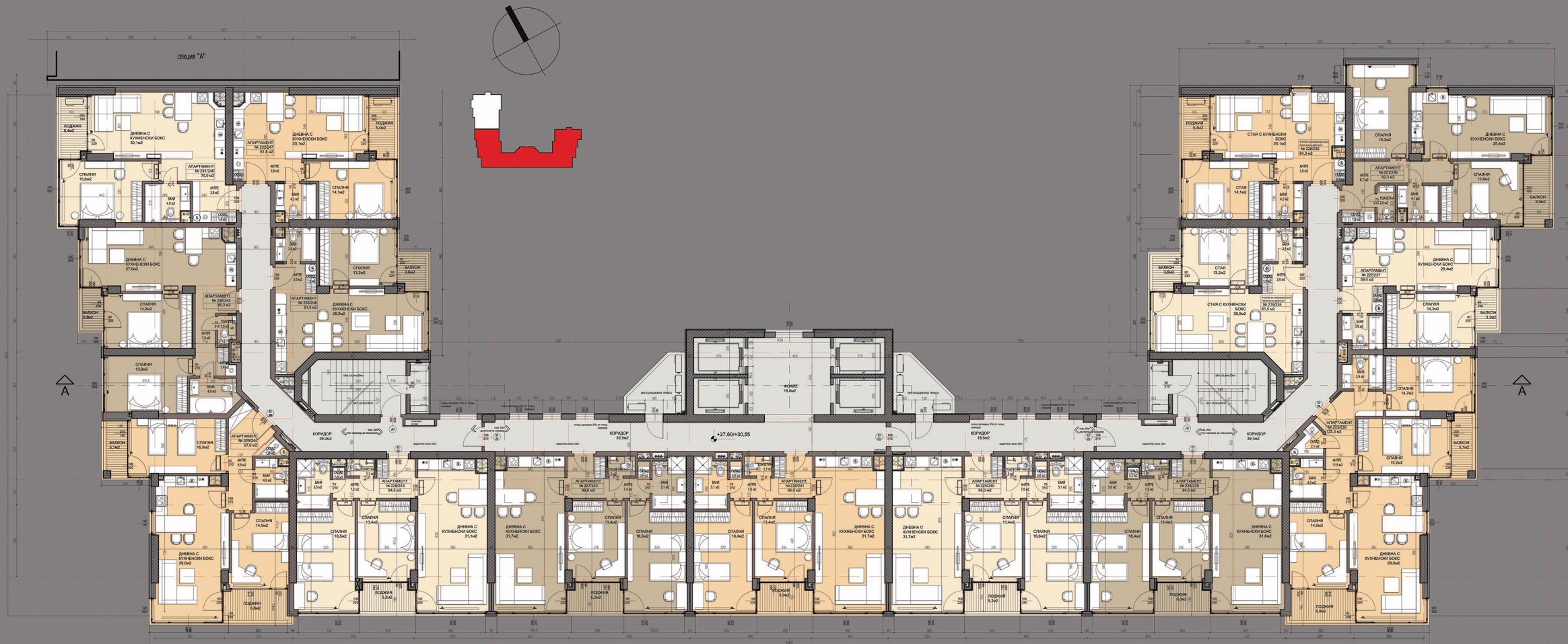
РАЗПРЕДЕЛЕНИЕ 10,11 ЕТАЖ СЕКЦИЯ Б
