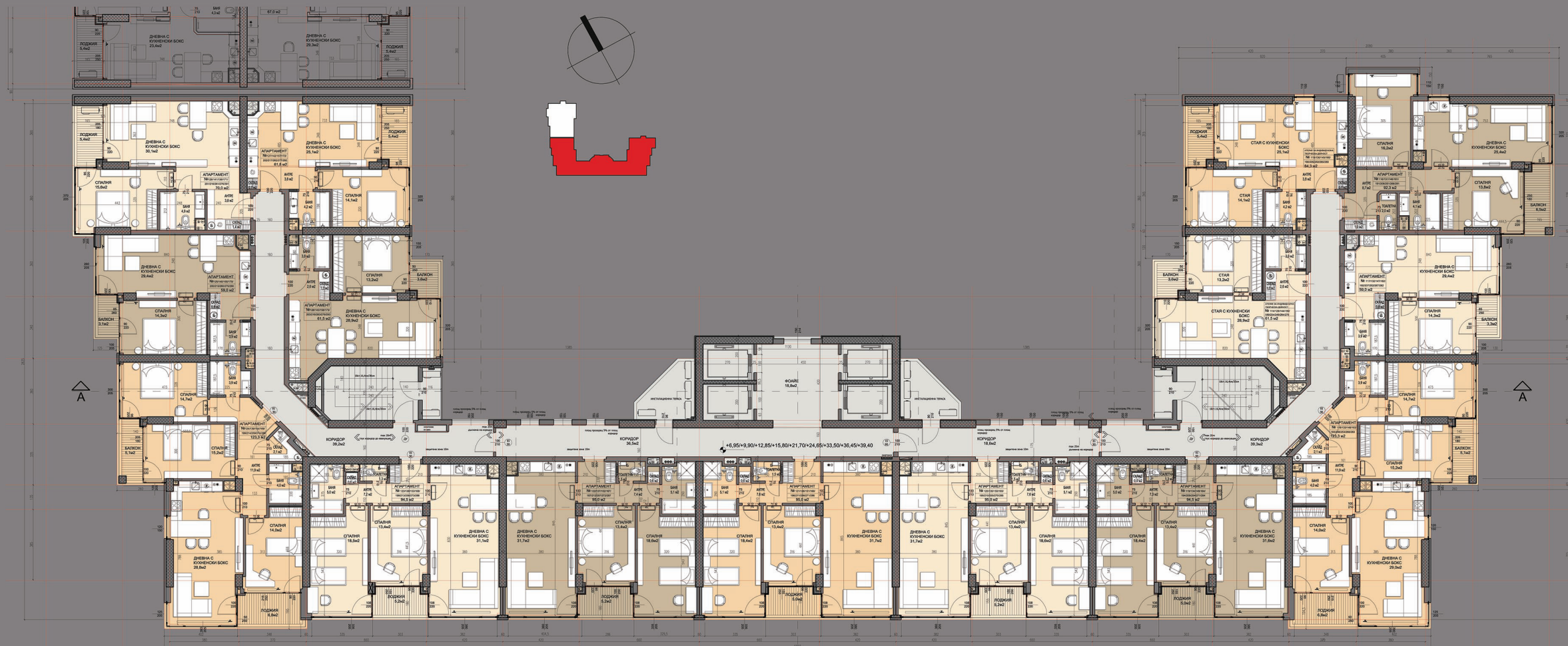
РАЗПРЕДЕЛЕНИЕ 3,4,5,6,8,9,12,13,14 ЕТАЖ СЕКЦИЯ Б
