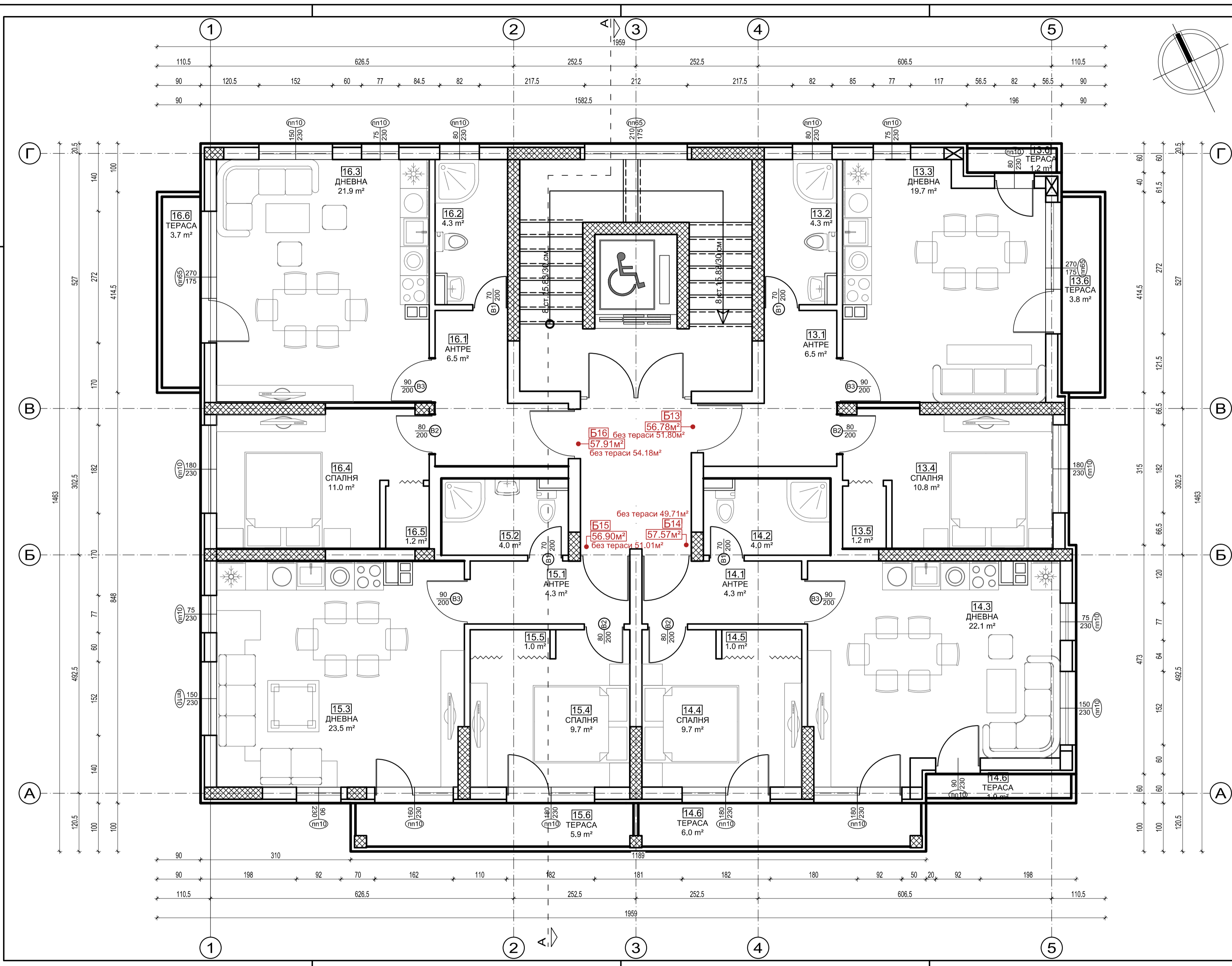
РАЗПРЕДЕЛЕНИЕ 4 ЕТАЖ 263.9 м²
