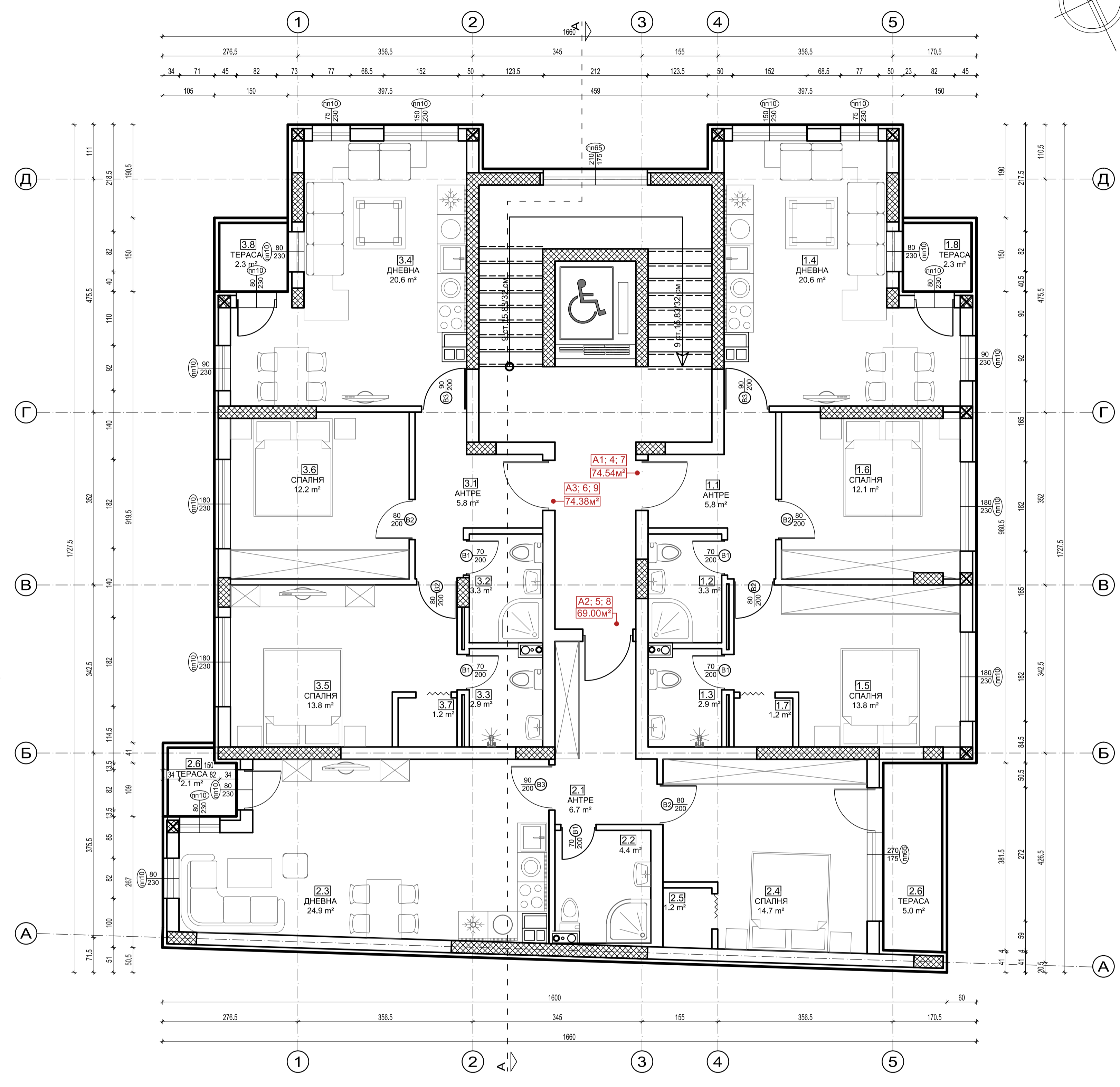
РАЗПРЕДЕЛЕНИЕ 2.3.4 ЕТАЖ 256.9 м2
