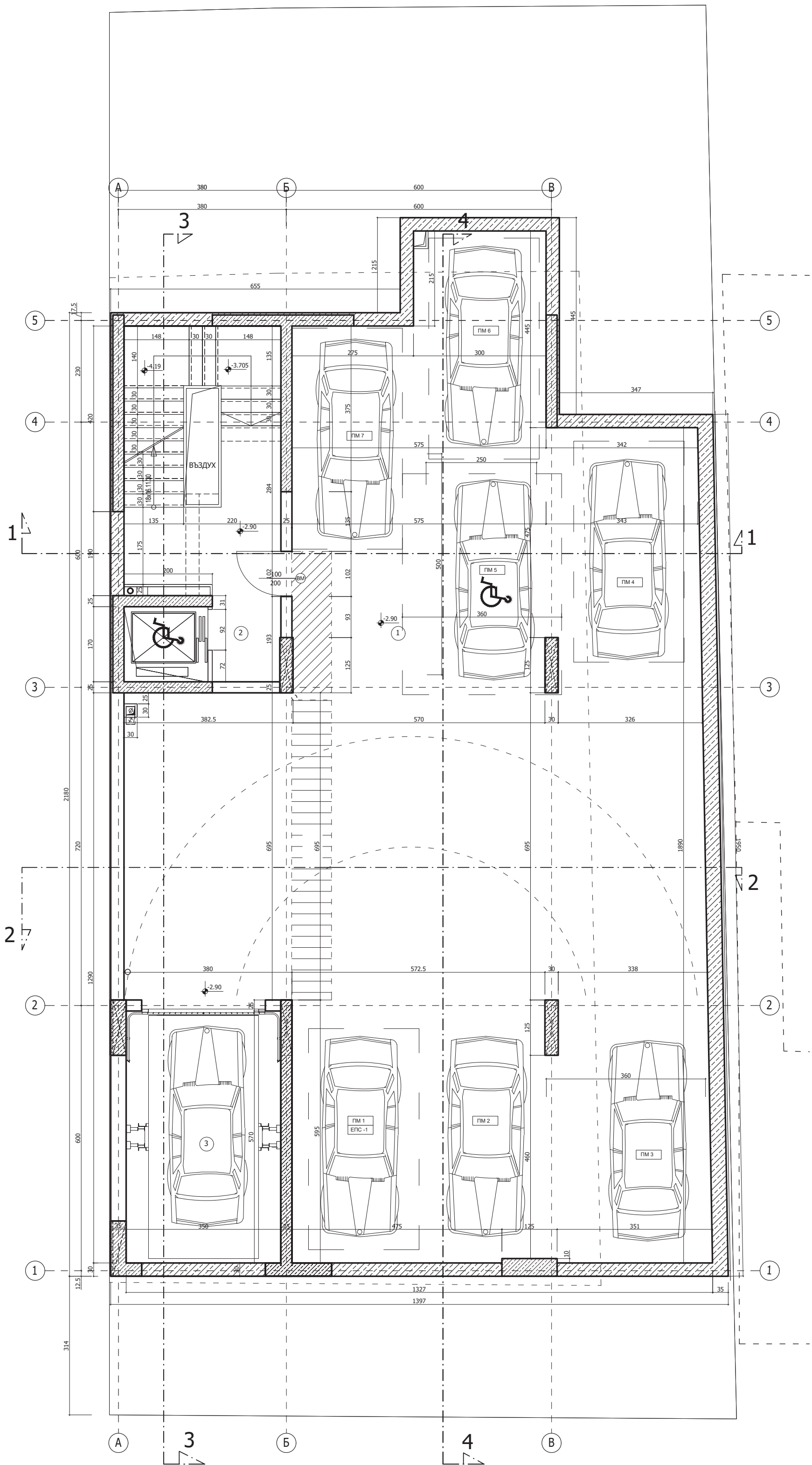
РАЗПРЕДЕЛЕНИЕ КОТА -2.90
