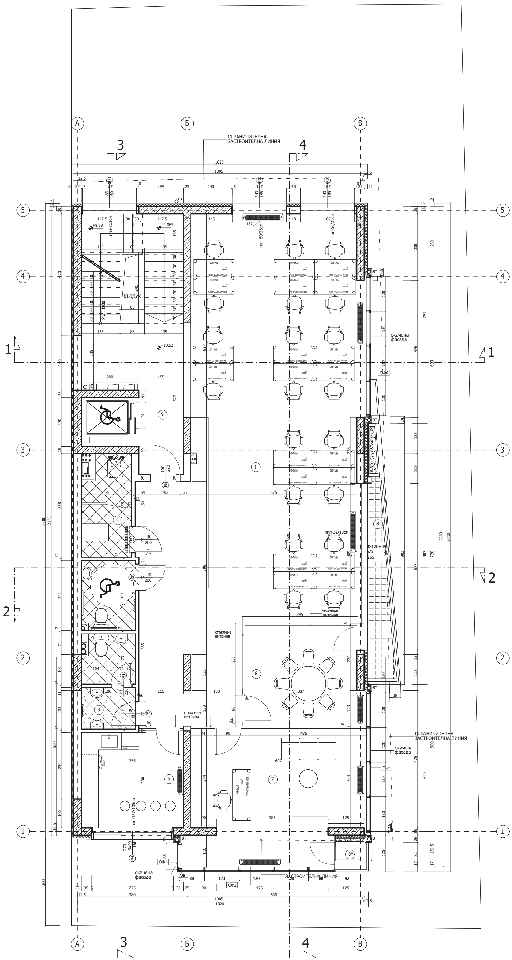
РАЗПРЕДЕЛЕНИЕ КОТА +10.52
