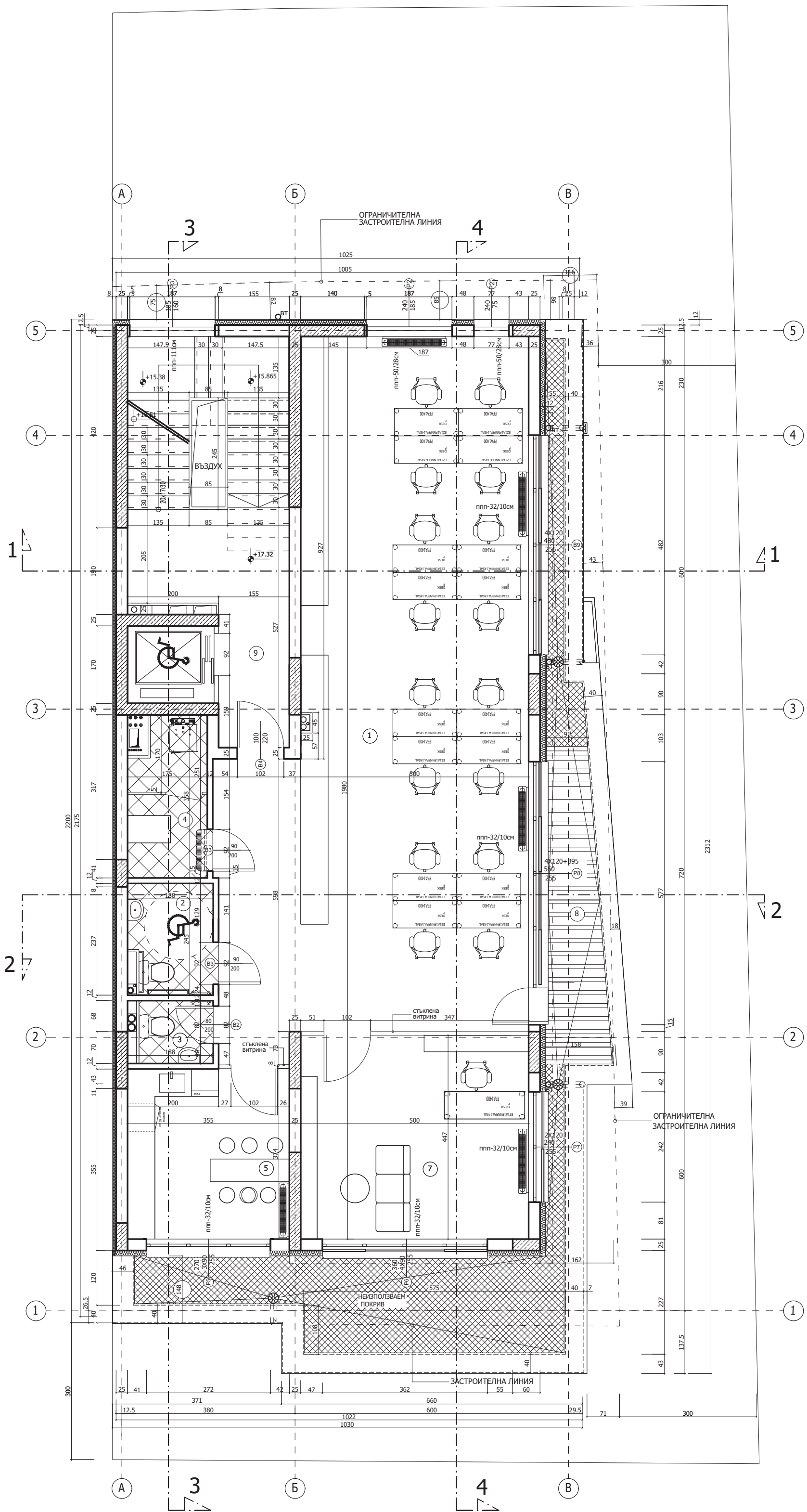
РАЗПРЕДЕЛЕНИЕ КОТА +17.32
