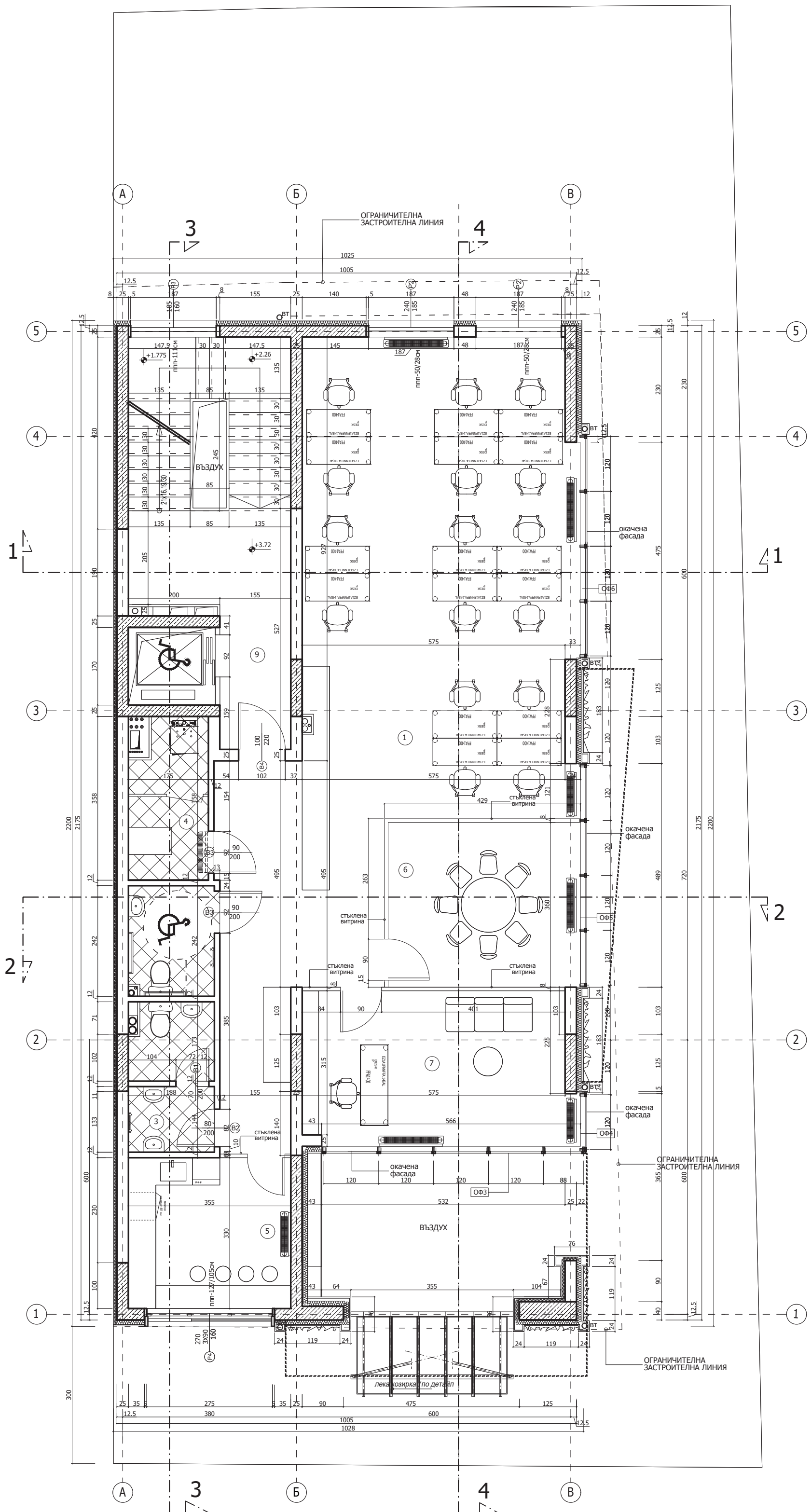
РАЗПРЕДЕЛЕНИЕ КОТА +3.72
