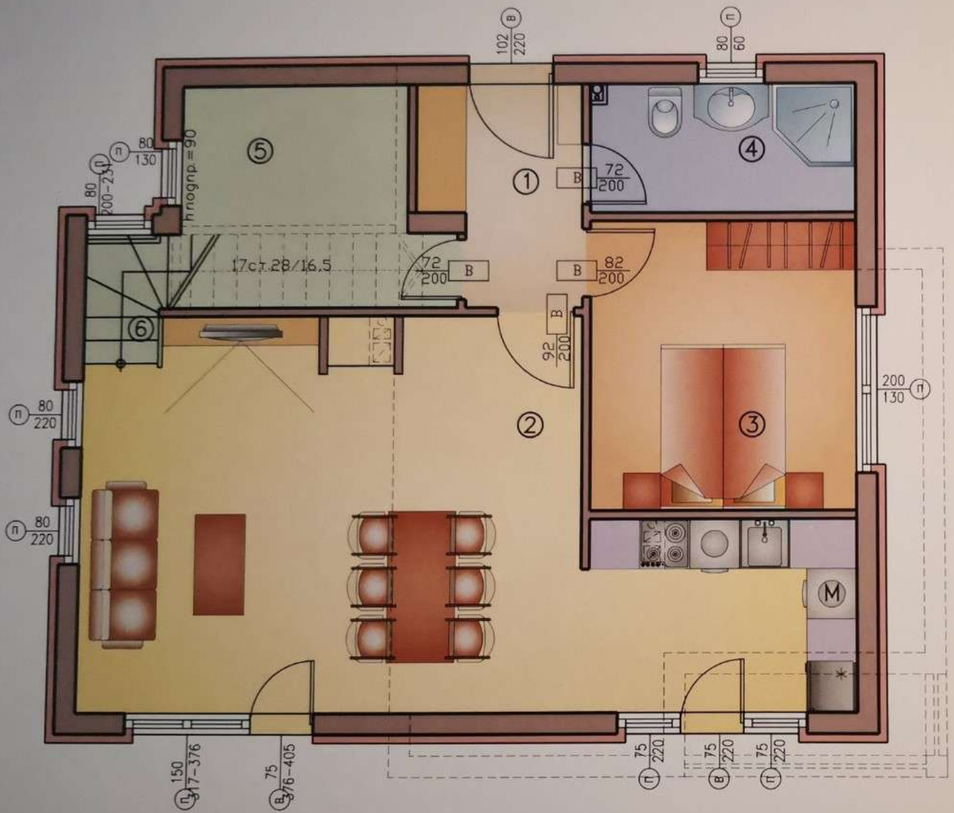
РАЗПРЕДЕЛЕНИЕ КОТА ±0.00 М 1:50
