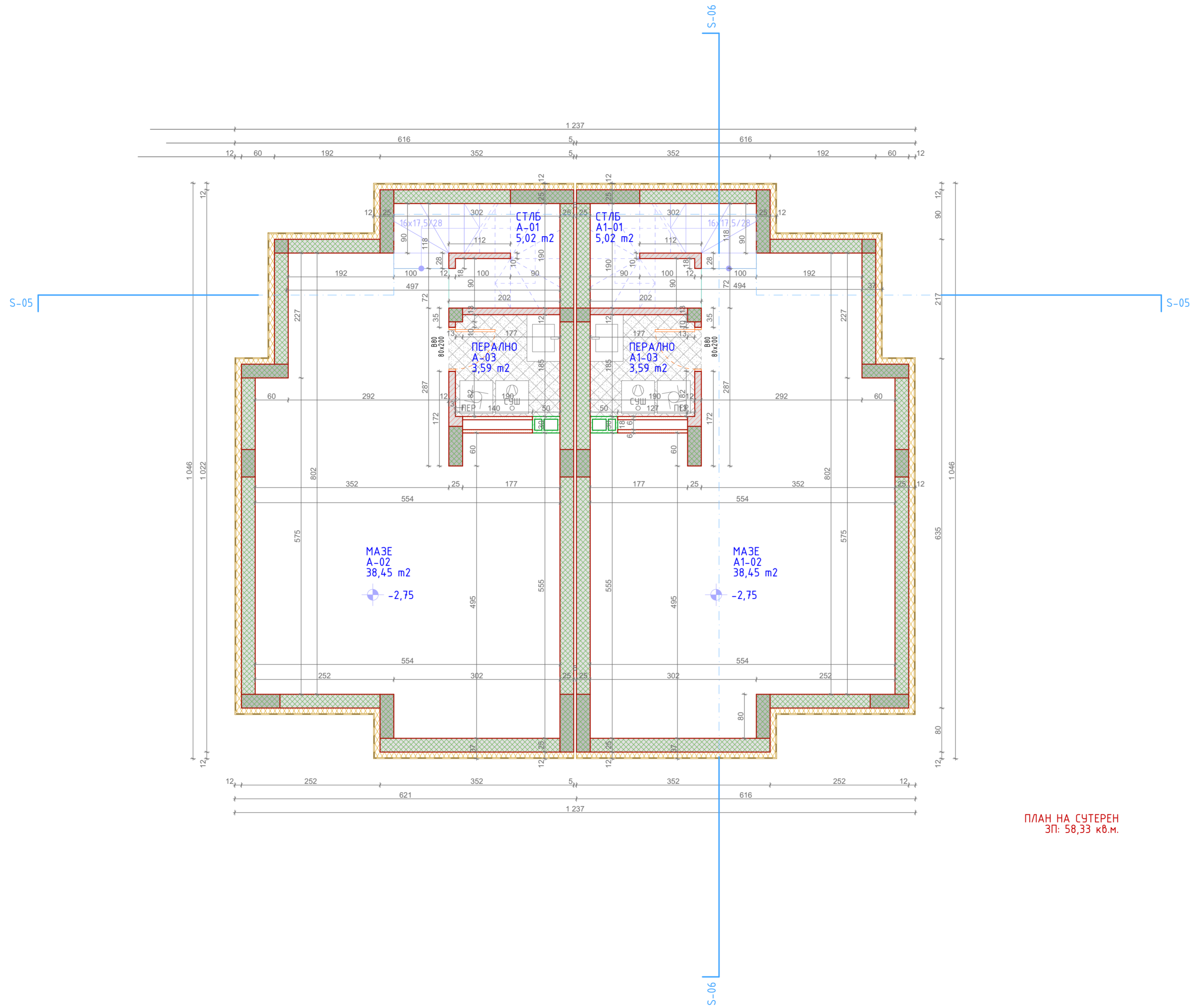
РАЗПРЕДЕЛЕНИЕ КЪЩИ А-А1 М 1:50
